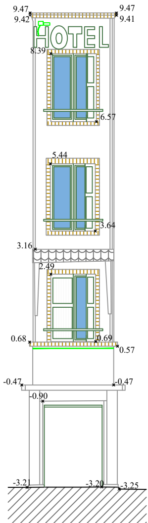
0 1 2 4 Façade-02
