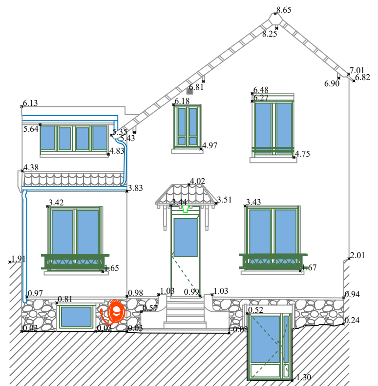
0 1 2 4 6 8 10 Façade-02
