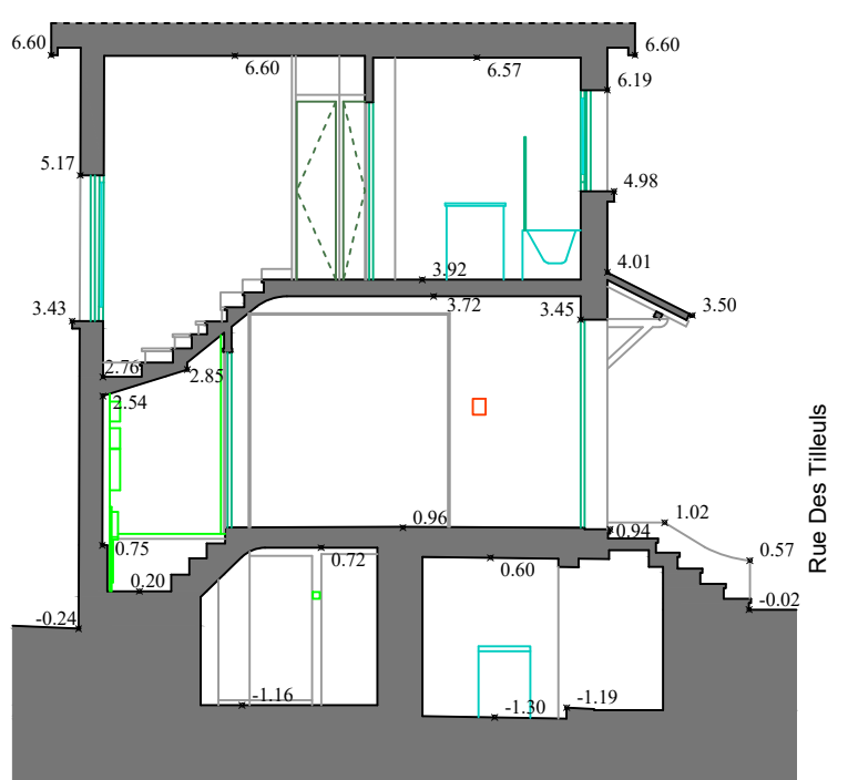
0 1 2 4 6 8 10 Coupe B-B
