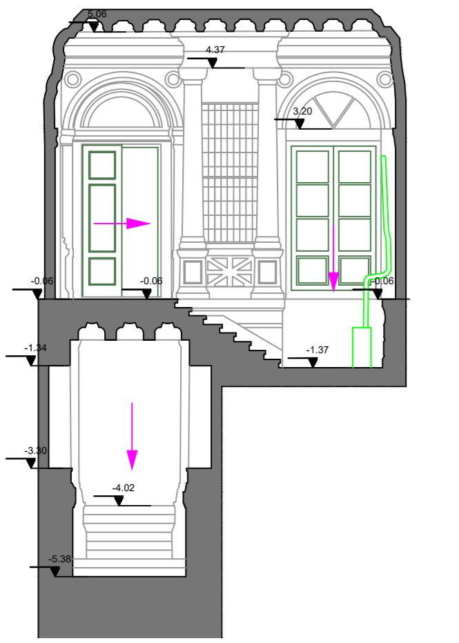
0 1 2 4 6 8 Coupe D-D
