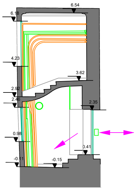
0 1 2 4 Coupe A-A
