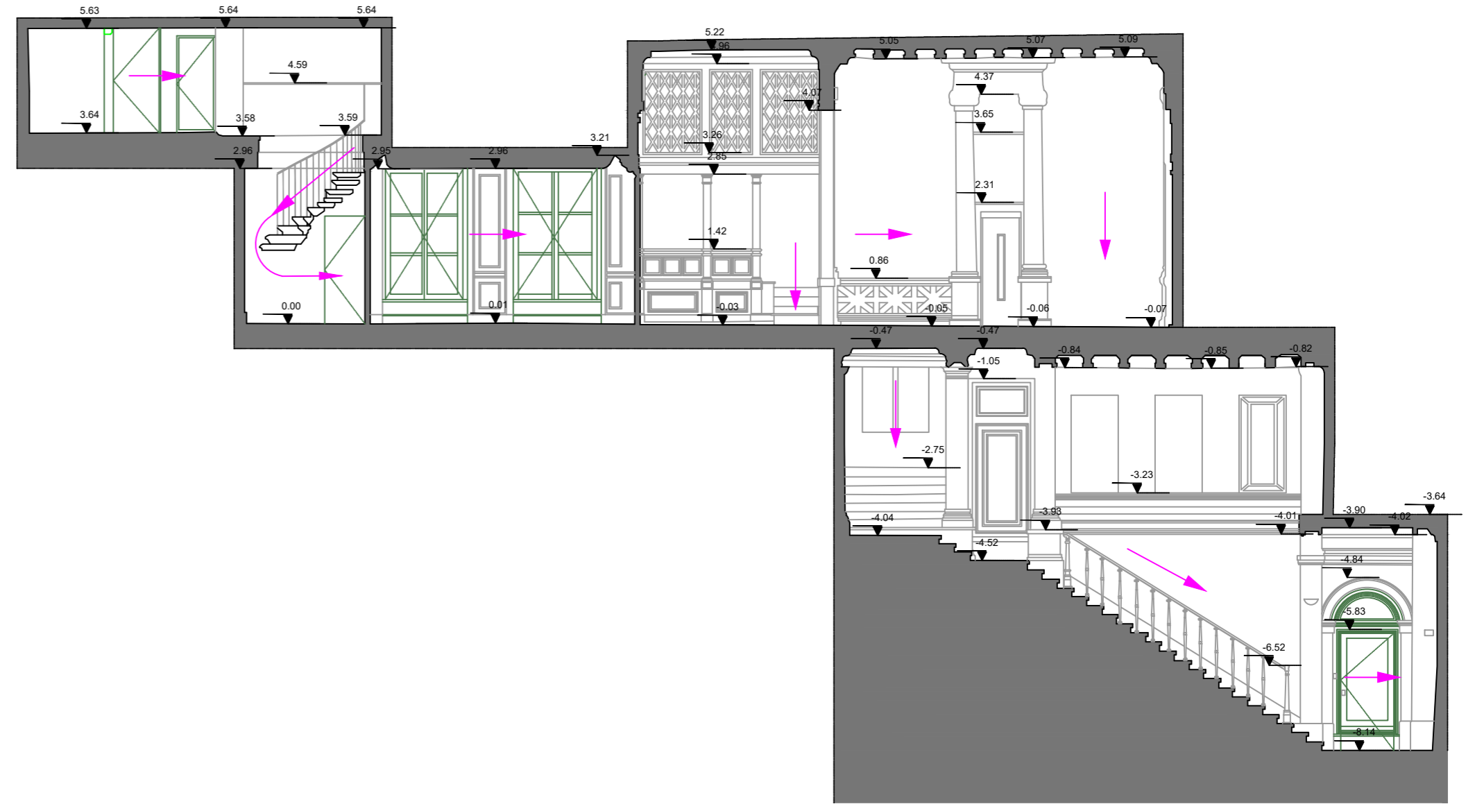
0 1 2 4 6 8 10 15 20 25 30 Coupe C-C
